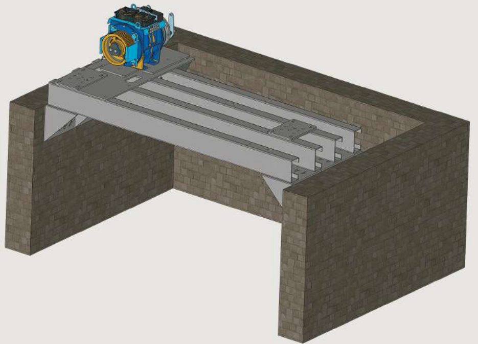
makine sehpası MRL DiSLiSİZ TİP 3 MR GEARLESS TYPE 3
