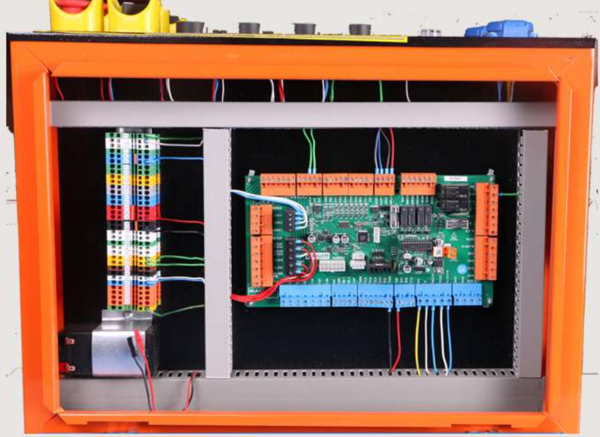
revizyon seti (revision set)
